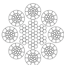
8XK26WS+IWRC R.1960N/mm 2
