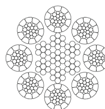
8XK26WS+IWRC R.2160N/mm 2
