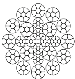
Non rotating 24xK7 2160N/mm 2
