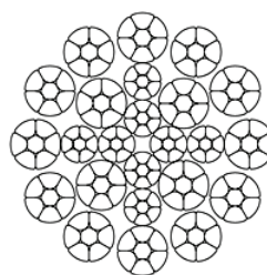
Non rotating 24xK7 1960N/mm 2
