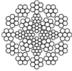
Non rotating 24x7 2160N/mm 2
