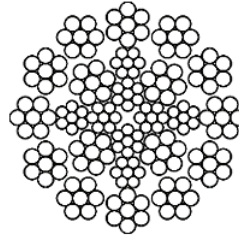
Non rotating 24x7 1960N/mm 2
